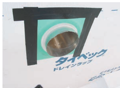
透湿防水シート及びサッシ・設備取合の確認
